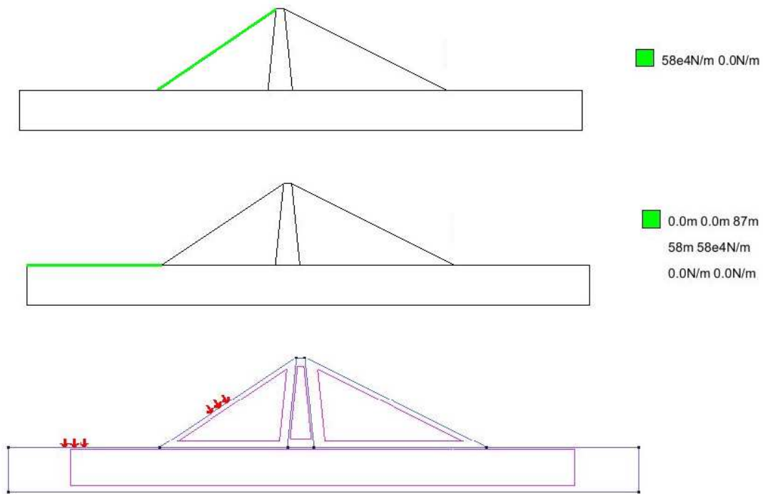
Figura 6. Introducción del empuje hidrostático
