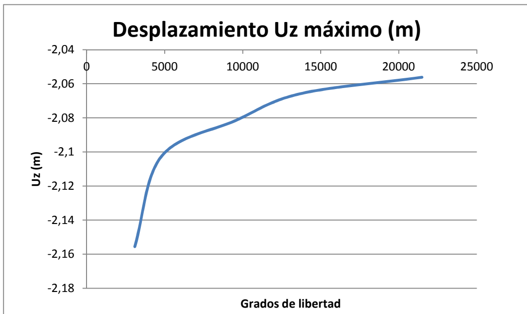
Figura 22. Análisis de convergencia del desplazamiento vertical
