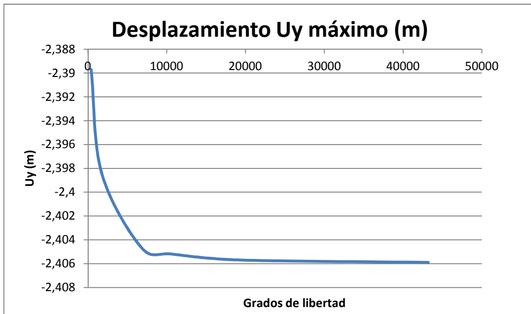
Figura 11. Análisis de convergencia del desplazamiento vertical
