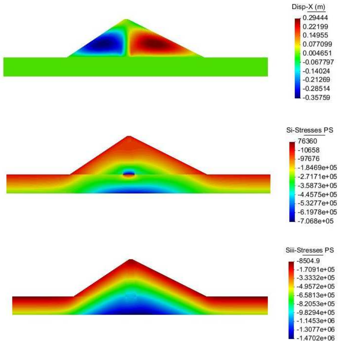
Figura 9. Resultados gráficos del campo de desplazamientos, de las tracciones (Si) y de las compresiones (Siii) para el caso 1
