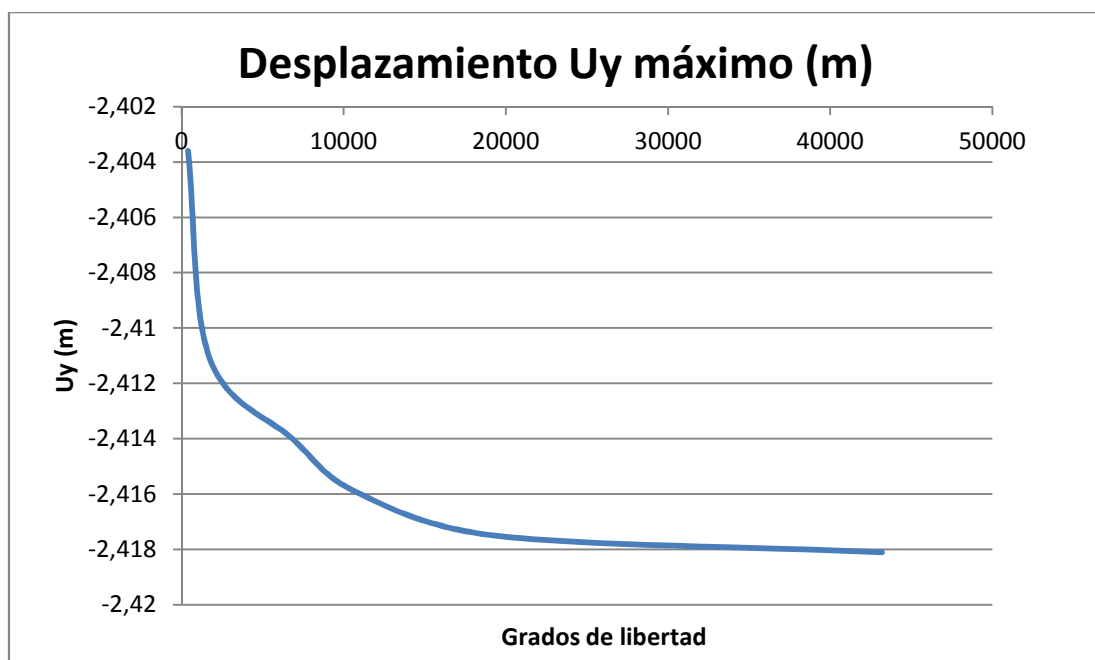
Figura 8. Análisis de convergencia del desplazamiento vertical
