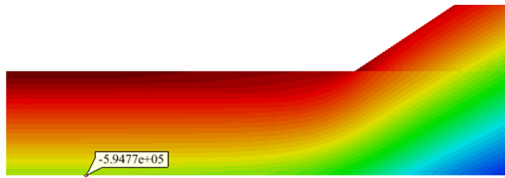
Figura 10. Compresión en la parte inferior del terreno
