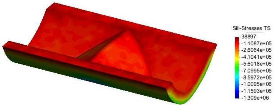
Figura 20. Resultados gráficos del campo de desplazamientos, de las tracciones (Si) y de las compresiones (Siii) para el caso 1
