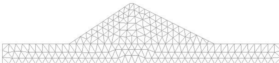
Figura 7. Ejemplo de malla utilizada
