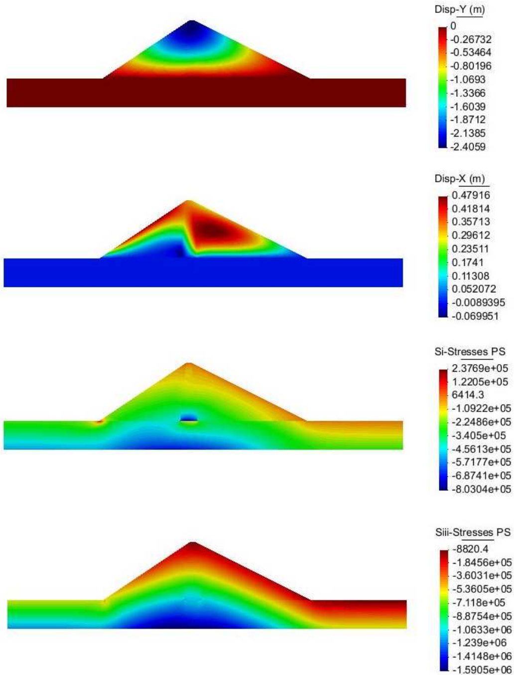
Figura 12. Resultados gráficos del campo de desplazamientos, de las tracciones (Si) y de las compresiones (Siii) para el caso 2
