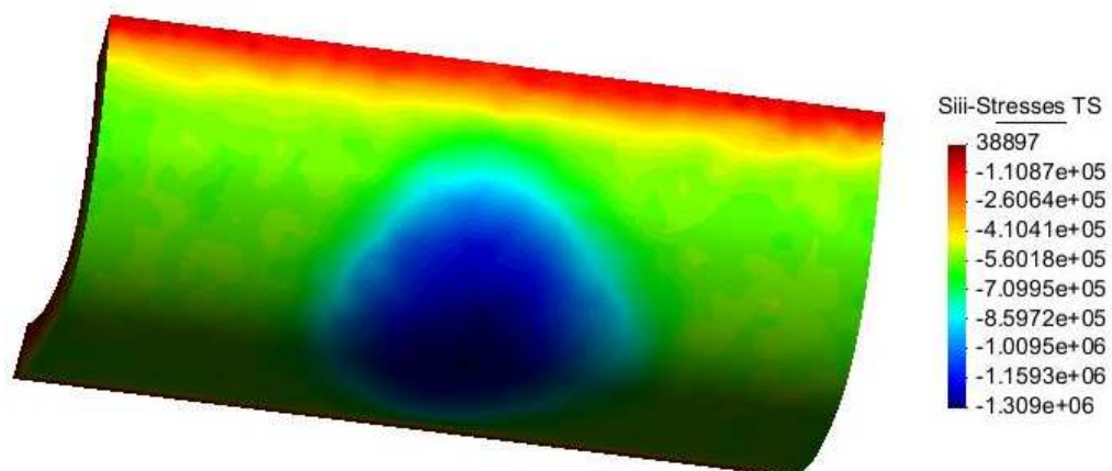
Figura 21. Compresiones en la base del terreno
