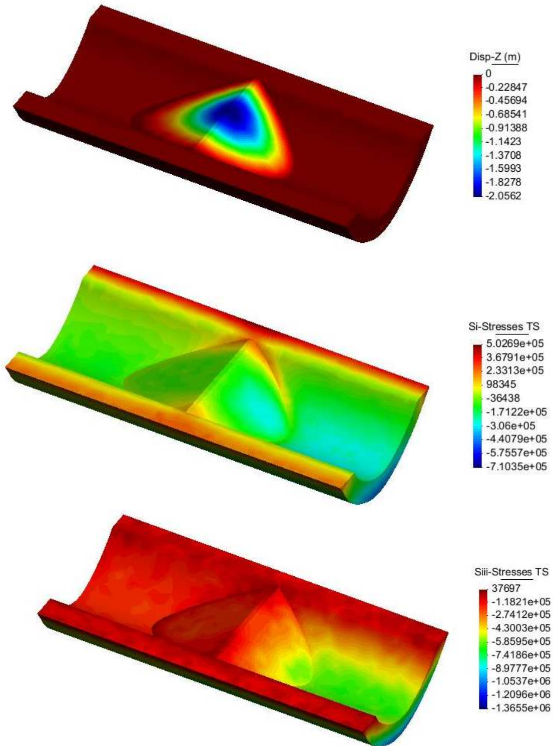
Figura 23. Resultados gráficos del campo de desplazamientos, de las tracciones (Si) y de las compresiones (Siii) para el caso 2
