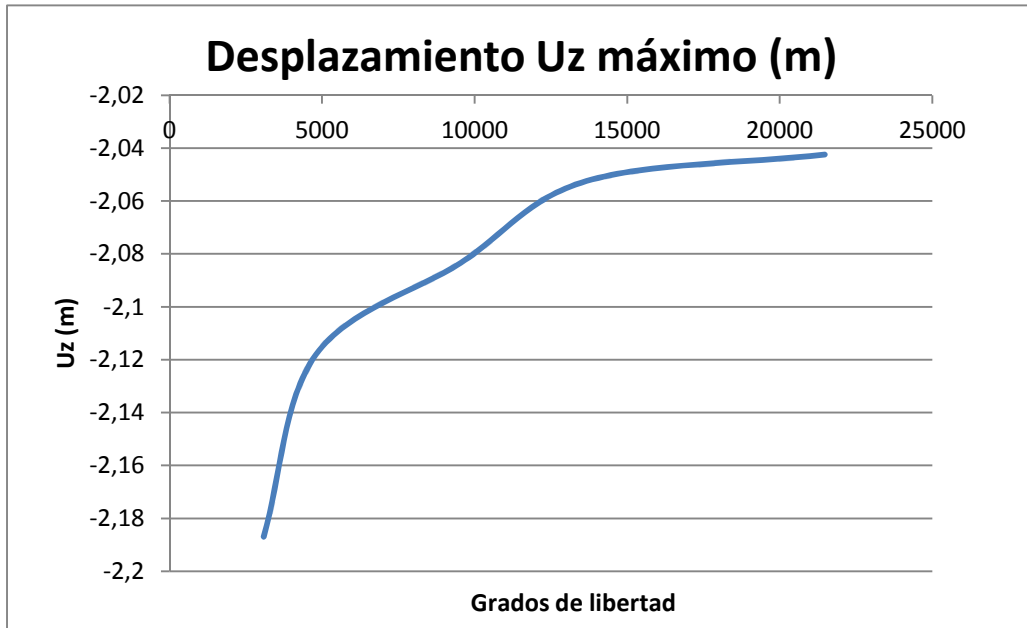
Figura 19. Análisis de convergencia del desplazamiento vertical
